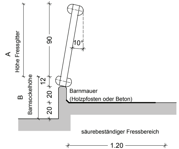
ANSICHT UND SCHNITT
