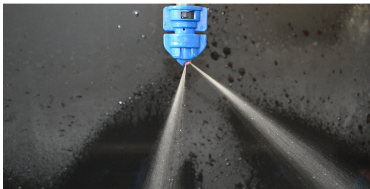
Asymmetrische Doppelfachstrahldüse
